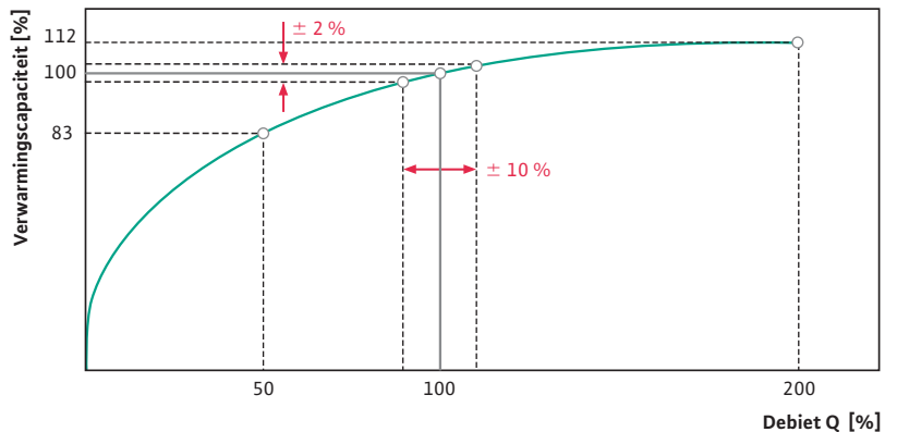
Radiator-bedrijfsdiagram
