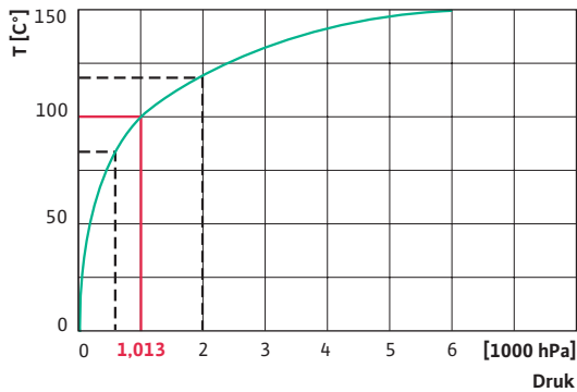
Kookpunt van water afhankelijk van de druk
